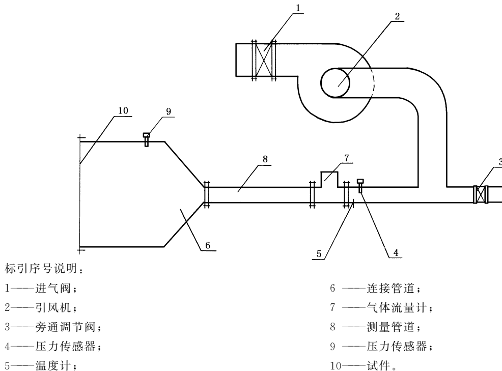
图 10 帘面漏烟量试验设备示意图
