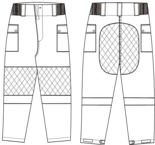
图A.2 夏款社区微型消防站训练服裤子正反面设计图
