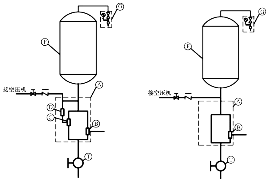
a) 机械式干式报警阀功能试验装置
