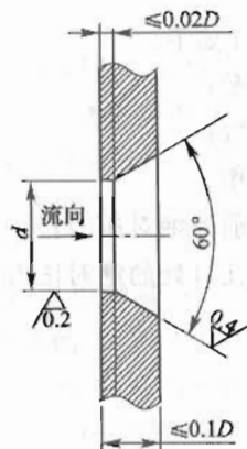
图 5 减压孔板
