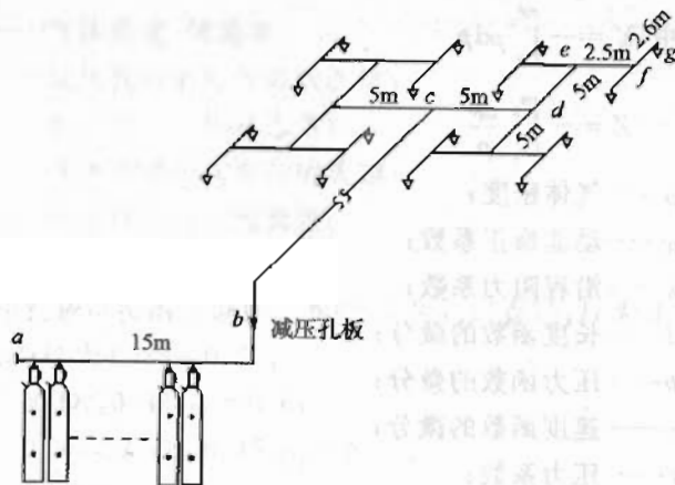
图6 系统管网计算图
