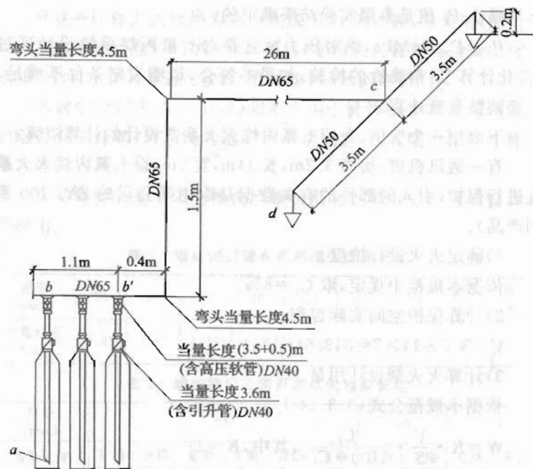
图 4 系统管网计算图
