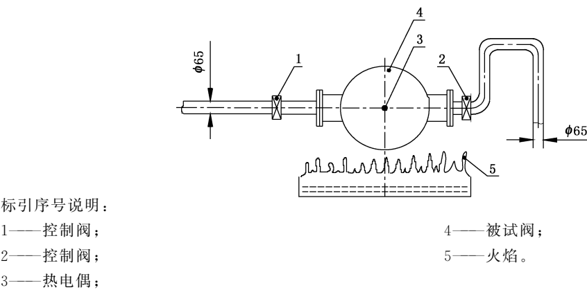
图 5 耐火试验布置
