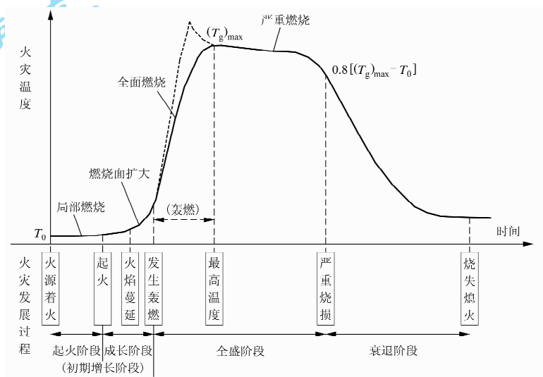
图 7 一般室内火灾的发展过程
