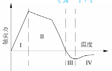
图 11 两端约束钢梁轴力随温度的变化图
