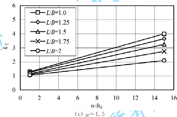
图 H.0.3 火灾下组合楼板考虑薄膜效应时的承载力增大系数 k_T
