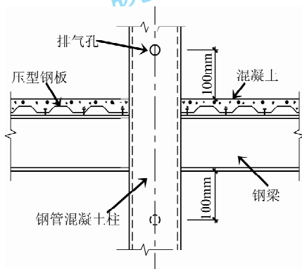
图 15 排气孔位置示意图
