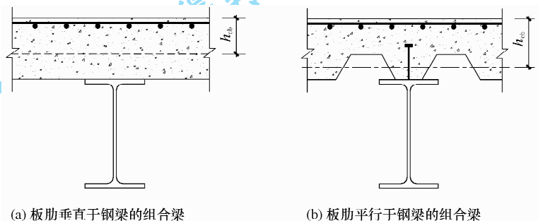
图 19 混凝土翼板的等效厚度 h_b
