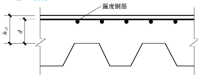
图 H.0.4 组合楼板的几何参数
