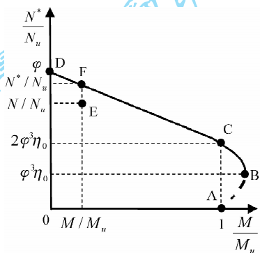
图 13 N^*/N_u - M/M_u 关系
