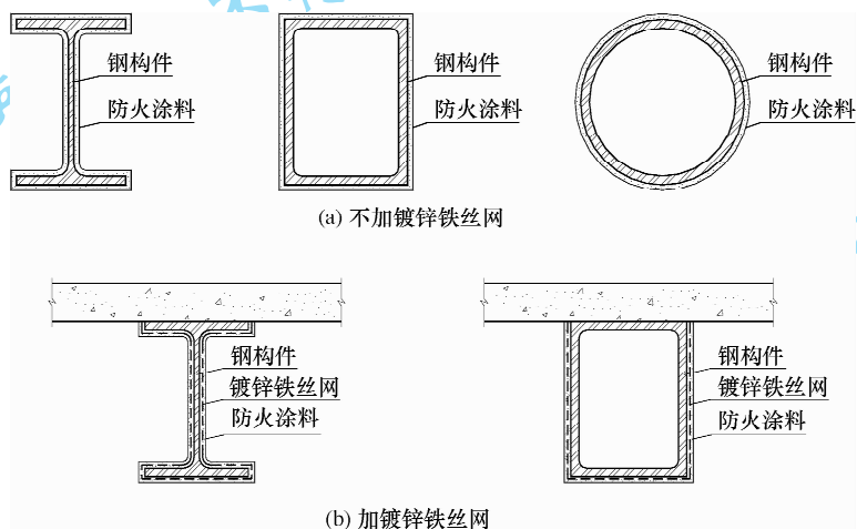
图 4.2.1 防火涂料的保护构造图
