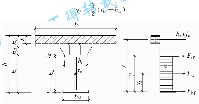
图 8.3.2-1 塑性中和轴在混凝土翼板内时组合梁截面的应力分布
