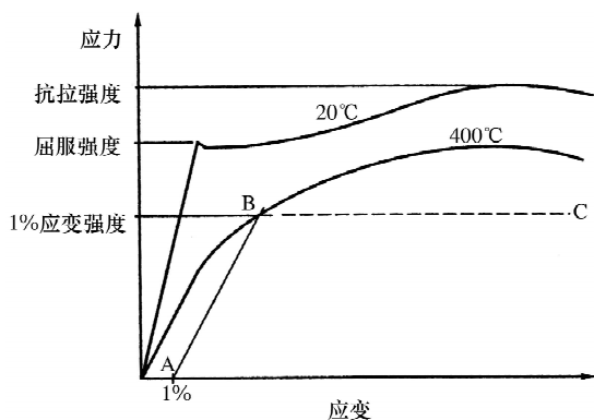
图 4 钢材高温名义屈服强度定义
