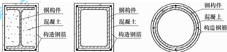
图 4.2.4 外包混凝土的防火保护构造图
