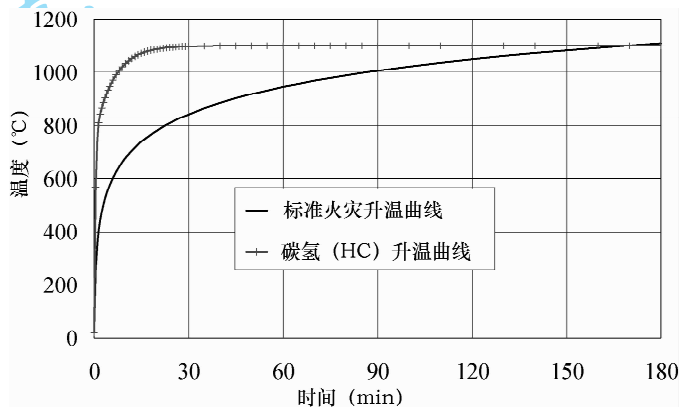
图 8 标准火灾升温曲线与碳氢(HC)升温曲线的比较
