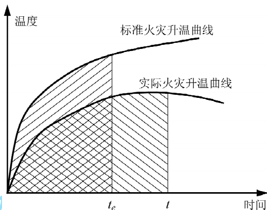
图 9 等效曝火时间 t_e
