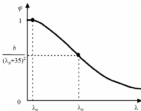
图 14 \varphi-\lambda 关系曲线示意图
