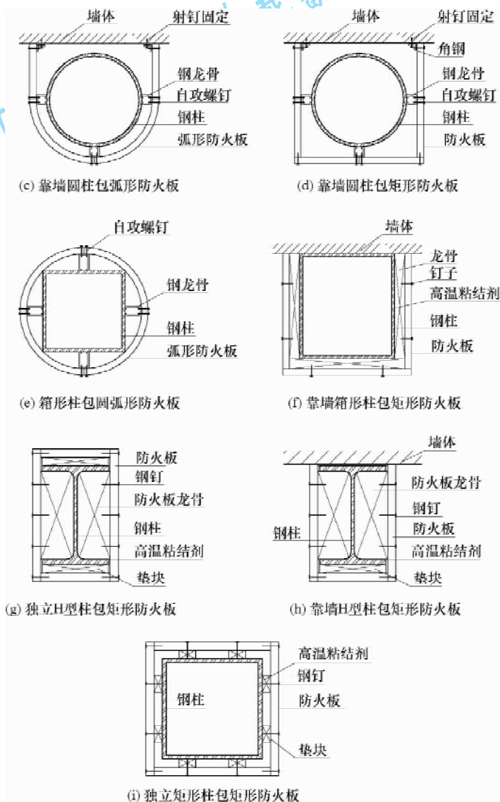
图 4.2.2-1 防火板保护钢柱的构造图
