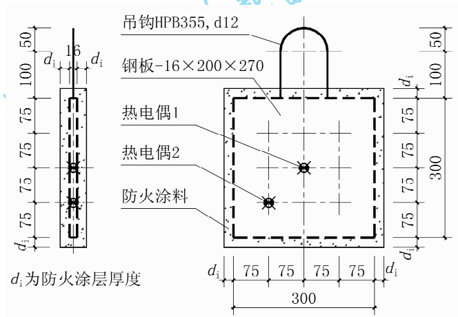
图 B.0.3 防火涂料等效热传导系数试件(单位:mm)
