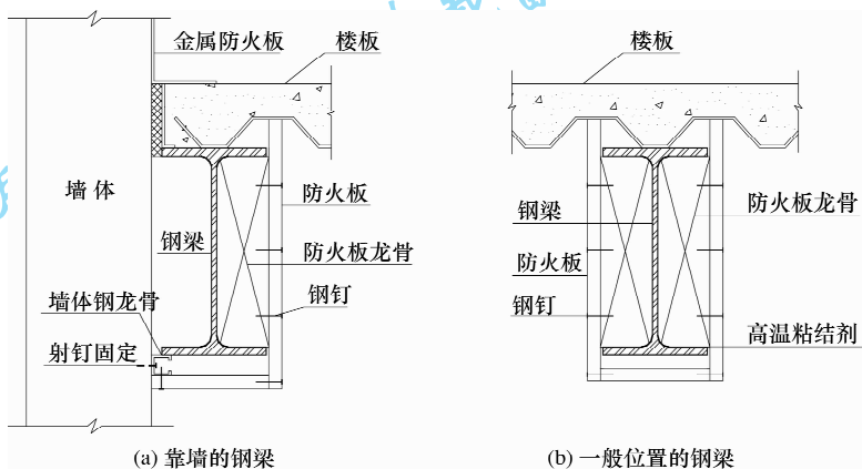
图 4.2.2-2 防火板保护钢梁的构造图
