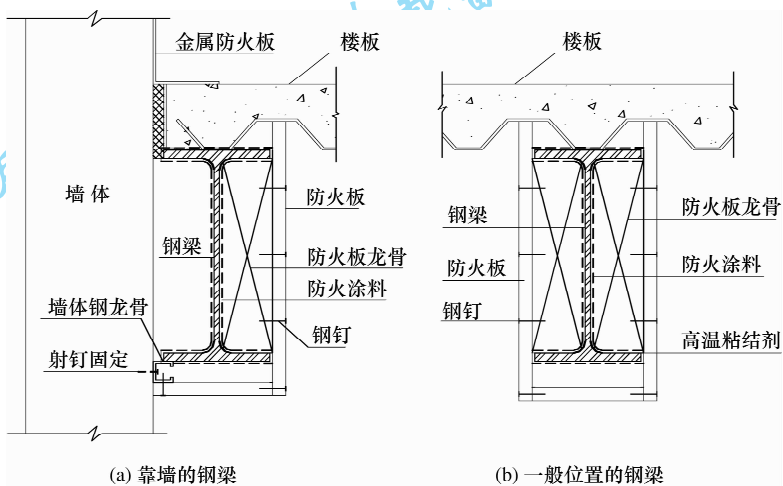
图 4.2.5-3 钢梁采用防火涂料和防火板复合保护的构造图
