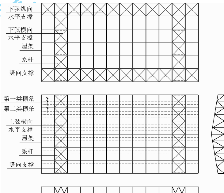
图 1 典型的屋盖结构体系
