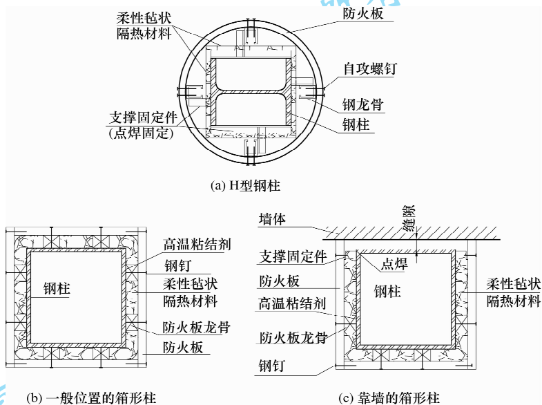
图 4.2.5-2 钢柱采用柔性毡和防火板复合保护的构造图
