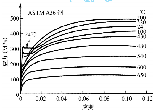
图 3 ASTM A36 钢的高温应力-应变曲线
