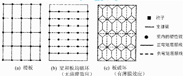
图 18 楼板弯曲破坏的形式
