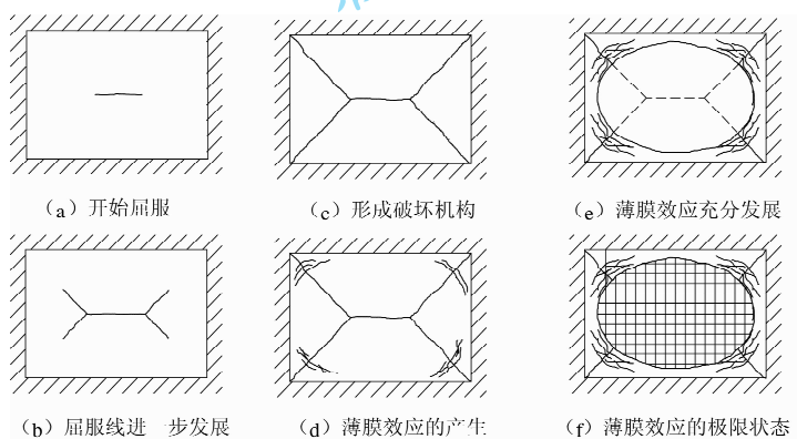
图 17 均匀受荷楼板随着温度升高形成薄膜效应的过程
