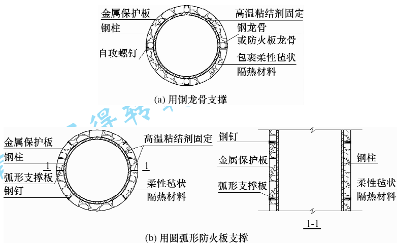
图 4.2.3 柔性毡状隔热材料的防火保护构造图
