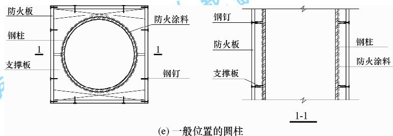
图 4.2.5-1 钢柱采用防火涂料和防火板复合保护的构造图
