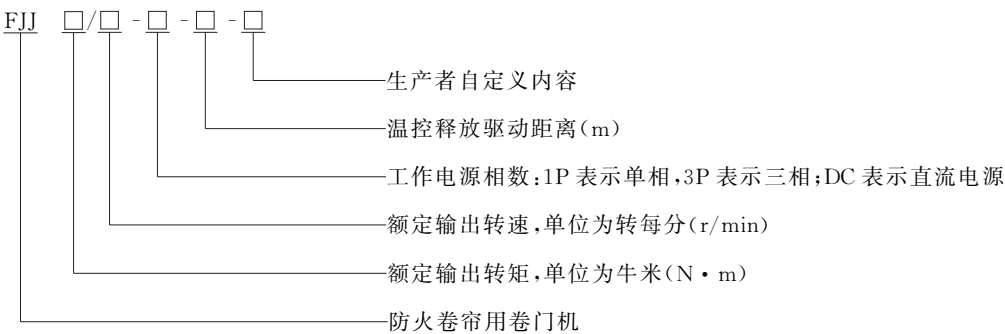
图 1 防火卷帘用卷门机型号编制
